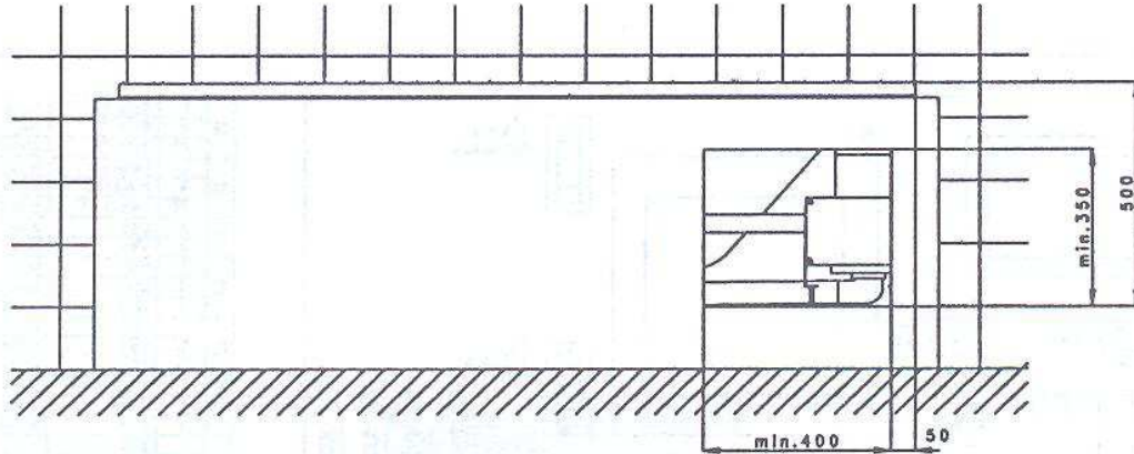
Erforderliche Revisionsöffnung
